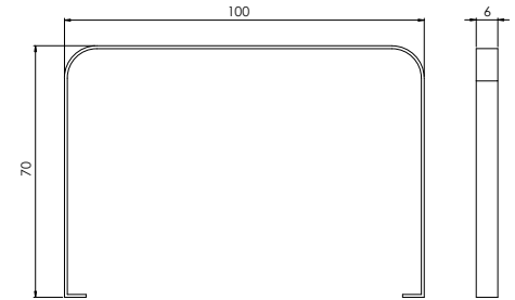
SC-K02 Opierky na bicykle Simplicity
