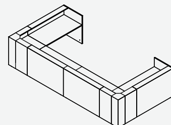
AS-REC-OL-80 2 ks Odporúčaný rozmer stola: AS-REC-EL-180 2 ks 2 ks 200 x 80 a AS-REC-SE-30 2 ks 2 ks 140 x 80 cm stôl AS-REC-EL-80 2 ks AS-REC-EL-140 2 ks 202/362/202 x 80 x 122 cm
