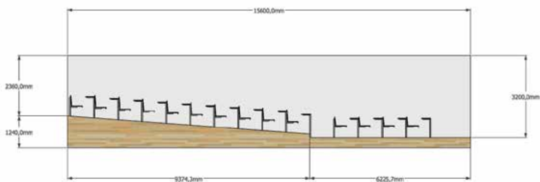
BOČNÝ POHĽAD
