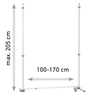
T-ÁLV-G Stojan na kolieskach
