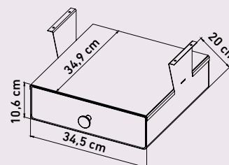
PF-35.10 PONTIS uzamykateľná zásuvka uzamykateľná, striekaný oceľový plech
